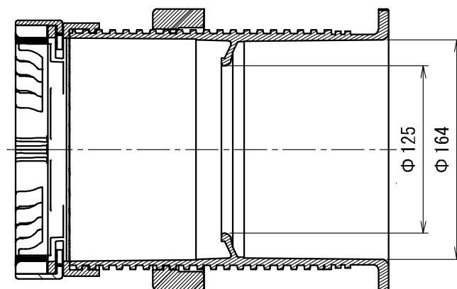
断面 A-A
